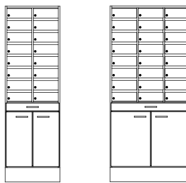
HPL2/16 605x1936x370
