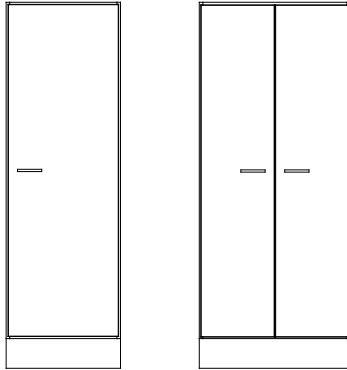
KL60 605x1936x570
